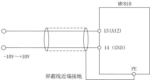
图 4-7 13 端子电压单端输入配线图
