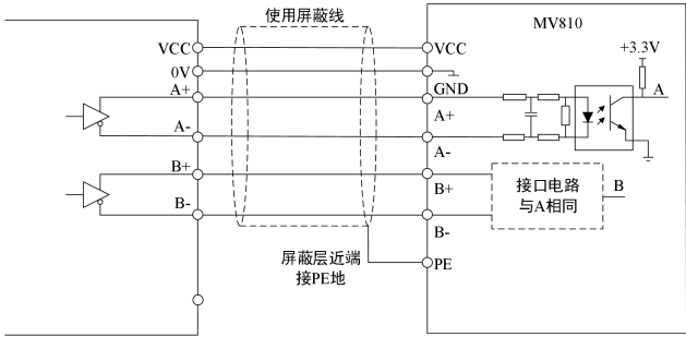
图 4-22 差分信号 PG 接线示意图
