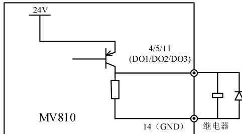
图 4-18 多功能输出端子 DO 接线方式
