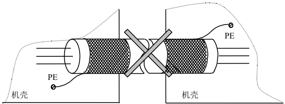
图 4-28 错误的屏蔽接地方法
