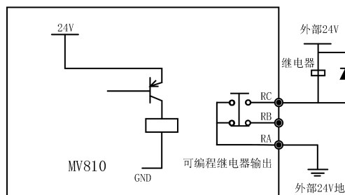
图 4-19 继电器输出端子 RA/RB/RC 接线方式
