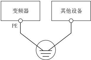
图 4-30 接地示意图 2
