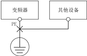
图 4-32 接地示意图 4
