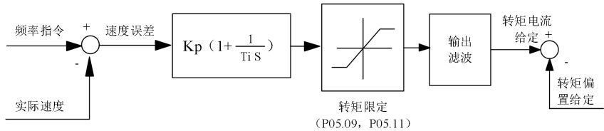
图7-10 速度调节器简化图
