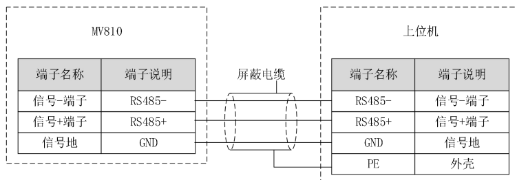
图 4-10 485-RS485 通讯配线
