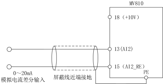
图 4-6 13 端子电流差分输入配线图
