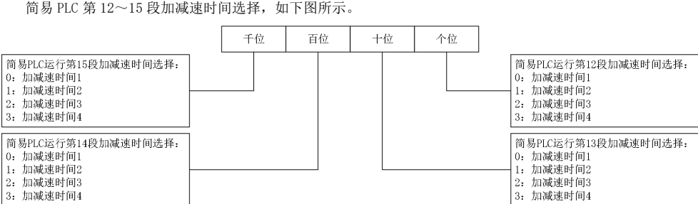
图7-43 简易PLC第12～15段加减速时间选择
