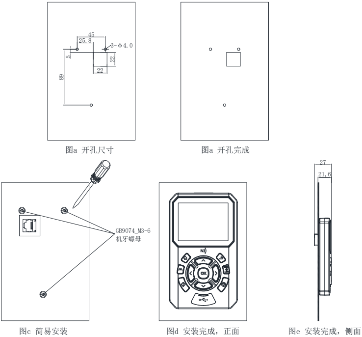
图2-51 大型远程LCD键盘/操作面板简易安装方法
