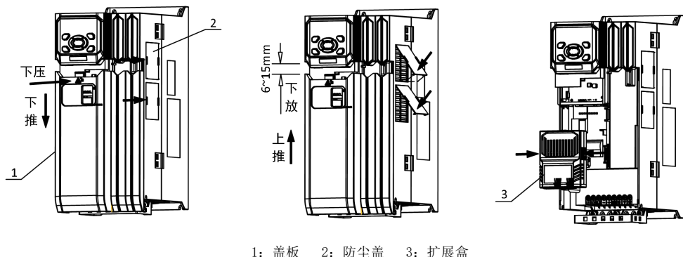
图 3-1 变频器部件的拆卸安装示意图（以箱体 C 为例）
