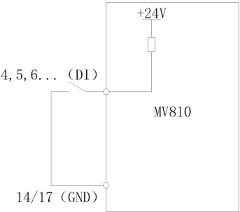
图 4-16 使用变频器内部+24V 电源连接方式
