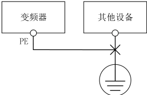
图 4-31 接地示意图 3
