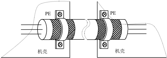
图 4-27 正确的屏蔽接地方法
