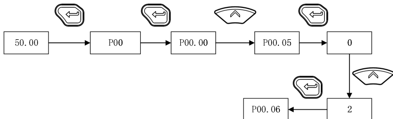
图 5-4 恢复出厂值设定操作示例
