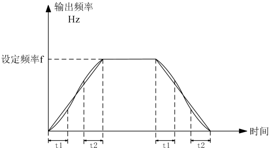
图7-28 S曲线开始、结束段时间比例
