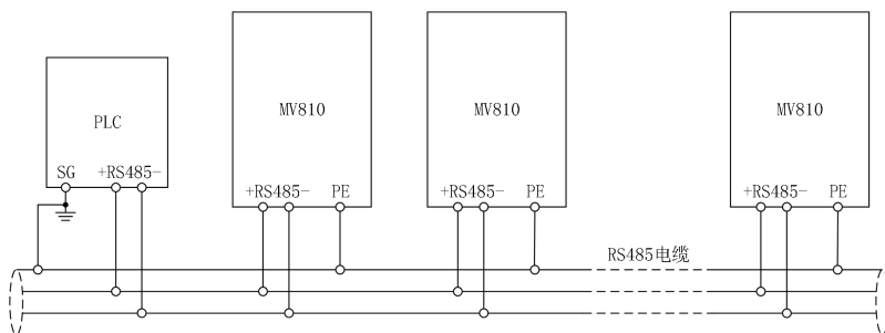
图 4-12 PLC 与变频器多机通讯时推荐的接线图（变频器、电机全部良好接地）
