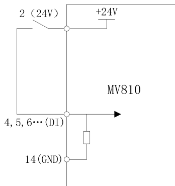
图 4-13 使用变频器内部+24V 电源连接方式
