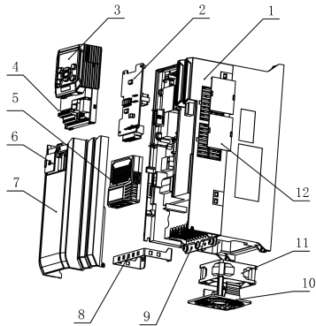
1：机箱 2：PG 卡 3：键盘 4：控制板 5：扩展盒 6：胶塞 7：上盖 8：绑线架 9：接地板 10：风扇罩 11：风扇 12：防静电板
