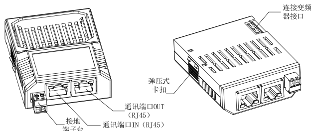
图2-9 端子部件示意图
