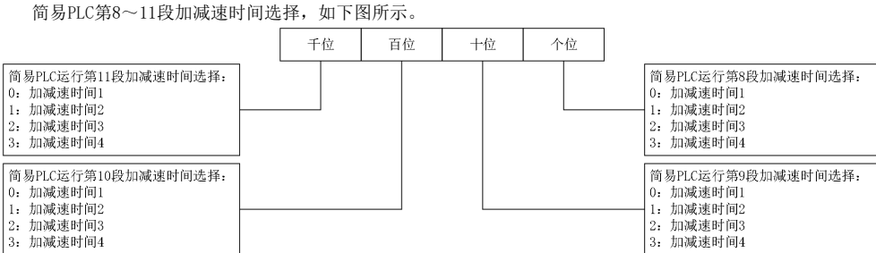
图7-42 简易PLC第8～11段加减速时间选择
