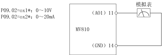
图 4-9 模拟输出端子配线
