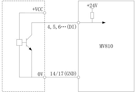
图 4-17 外部控制器为 NPN 连接方式
