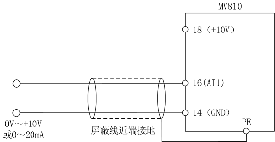
图 4-5 16 端子单端输入配线图
