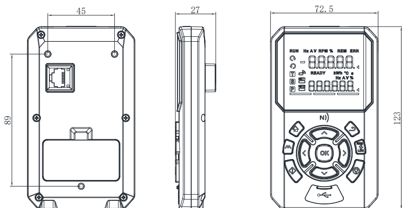
图2-48 大型远程LED键盘/操作面板 (单位: mm)
