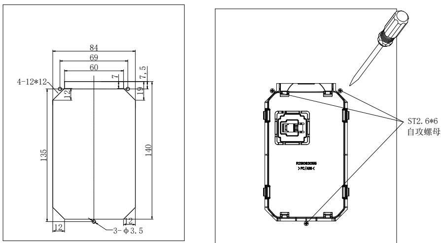
图2-45 大型操作面板固定座安装孔尺寸（单位：mm）
