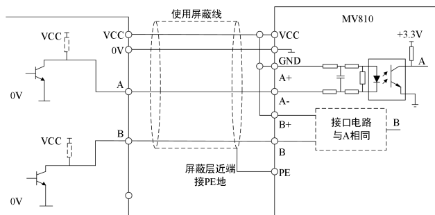
图 4-20 集电极开路信号 PG 接线示意图
