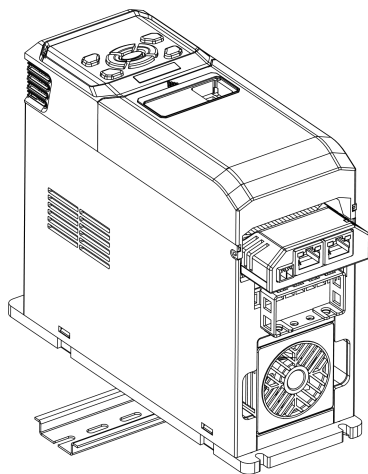
图 3-3 导轨式安装
