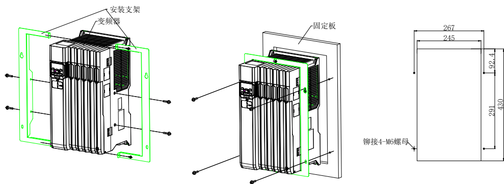
图2-37 MV810-EMBF (适用于30、37kW)
