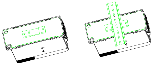
图2-41 轨道卡扣
