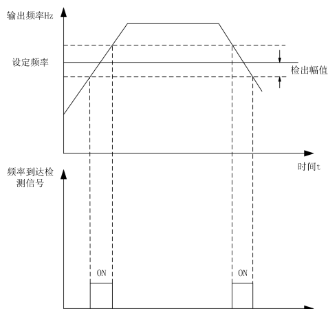
图7-32 频率到达 (FAR) 检出幅度
