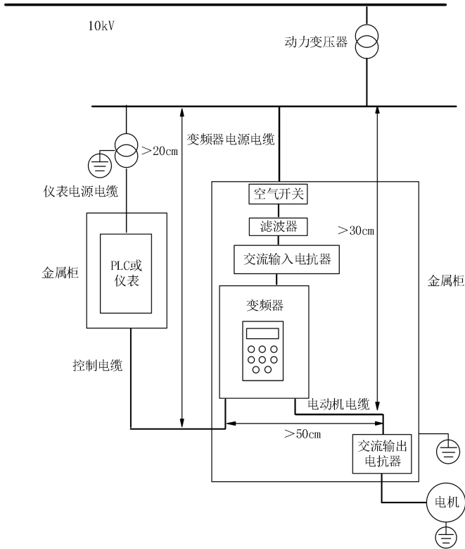
图 4-37 变频器的安装示意图
