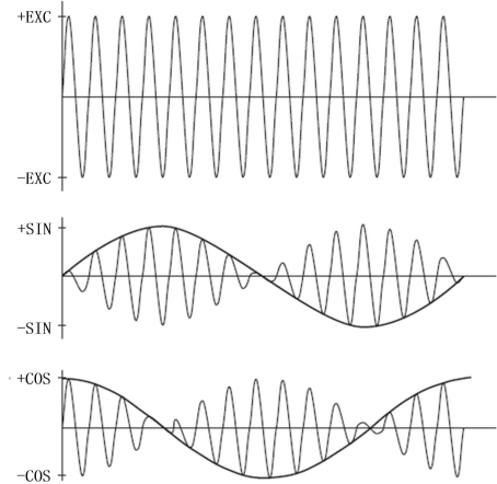
图2-27 旋变信号
