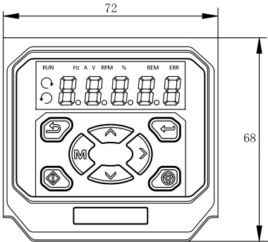
图 1-8 操作面板的外形和安装尺寸
