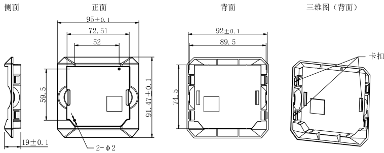
图2-42 键盘安装底座（单位：mm）
