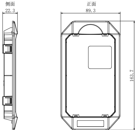
图2-44 大型键盘安装底座（单位：mm）
