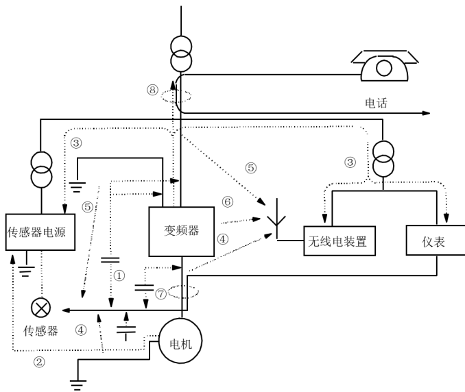
图 4-25 噪声传播路径示意图
