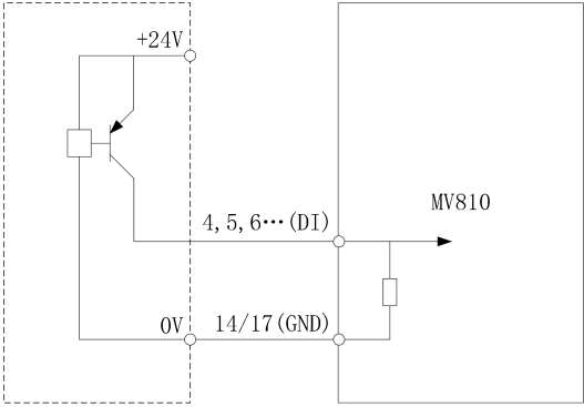
图 4-15 使用外部电源的 PNP 连接方式
