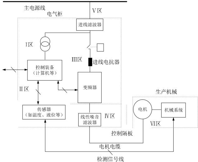
图 4-36 变频器 EMC 安装推荐区域划分示意图
