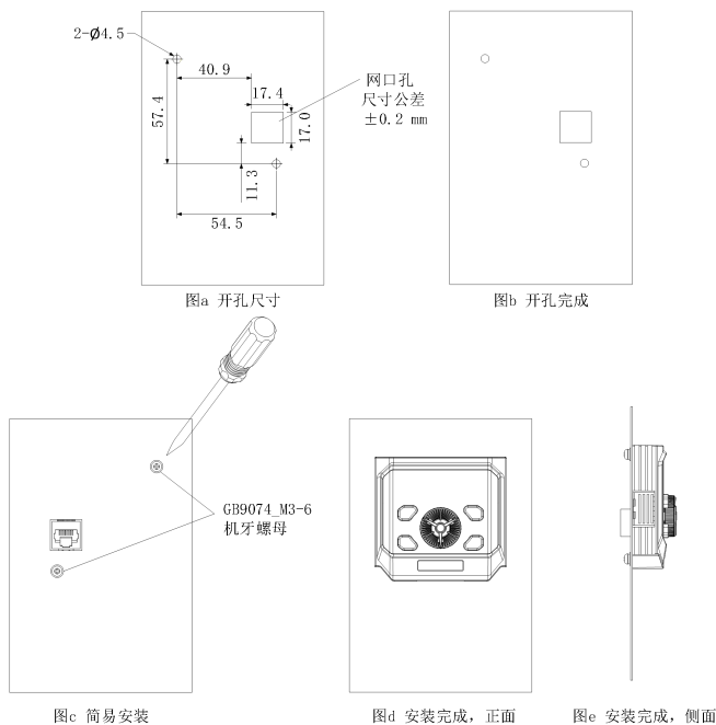
图2-47 远程LED键盘/操作面板简易安装方法
