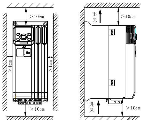
图 3-2 立式安装间隔距离
