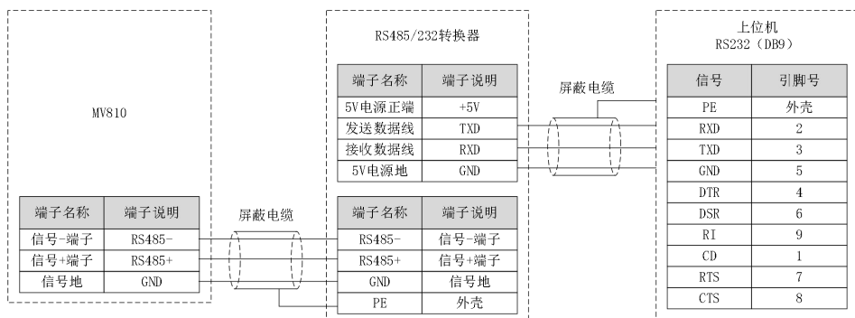
图 4-11 485-（RS485/232）-RS232 通讯配线
