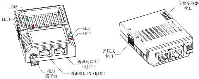
图2-32 产品外观
