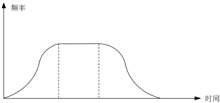
图7-27 S曲线加减速
