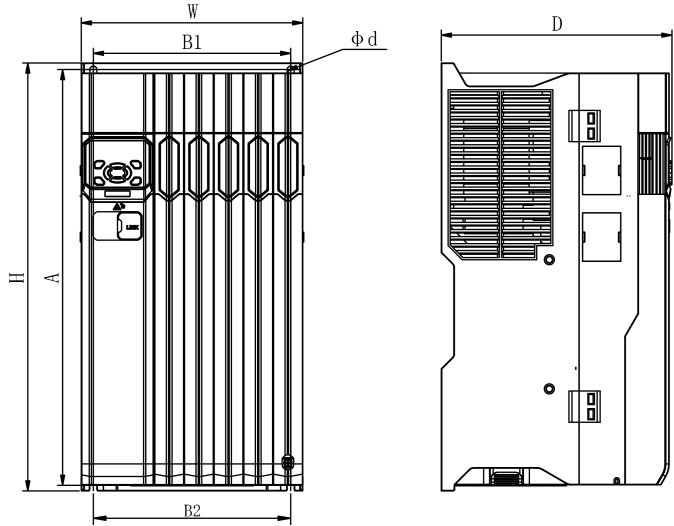
图 1-6 箱体 F
