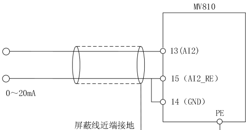
图 4-8 13 端子电流单端输入配线图
