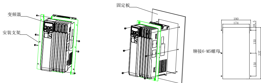
图2-36 MV810-EMBE (适用于18.5~22kW)
