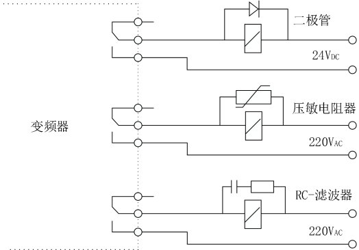
图 4-33 继电器、接触器及电磁制动器要求
