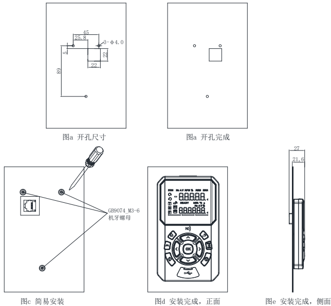
图2-49 大型远程LED键盘/操作面板简易安装方法
