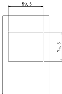
图2-43 操作面板固定座安装孔尺寸（单位：mm）
