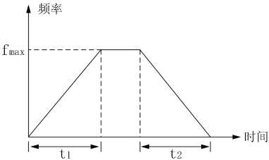
图7-26 直线加减速
