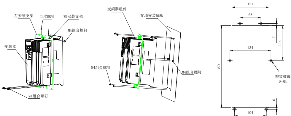
图2-34 MV810-EMBC (适用于5.5~7.5kW)
