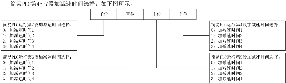
图7-41 简易PLC第4～7段加减速时间选择
