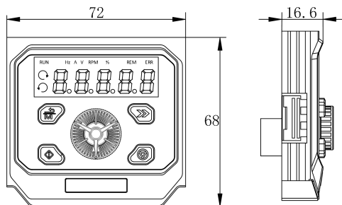
图2-46 小型远程LED键盘/操作面板
