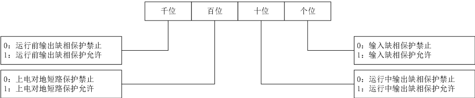
图7-51 输入、输出缺相保护设定
