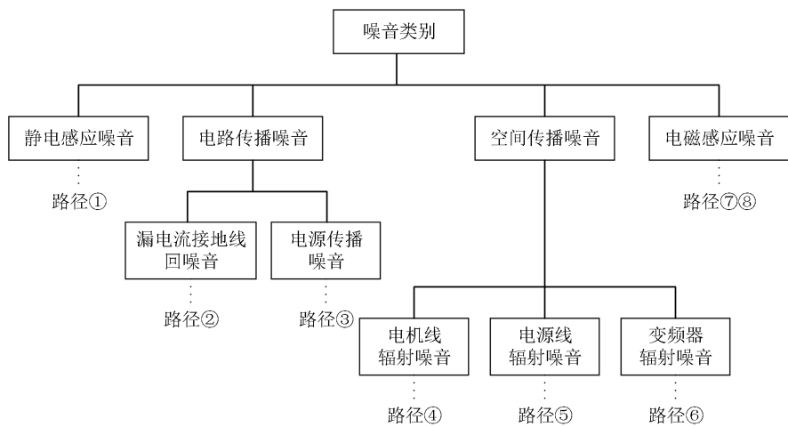
图 4-24 噪声分类示意图
