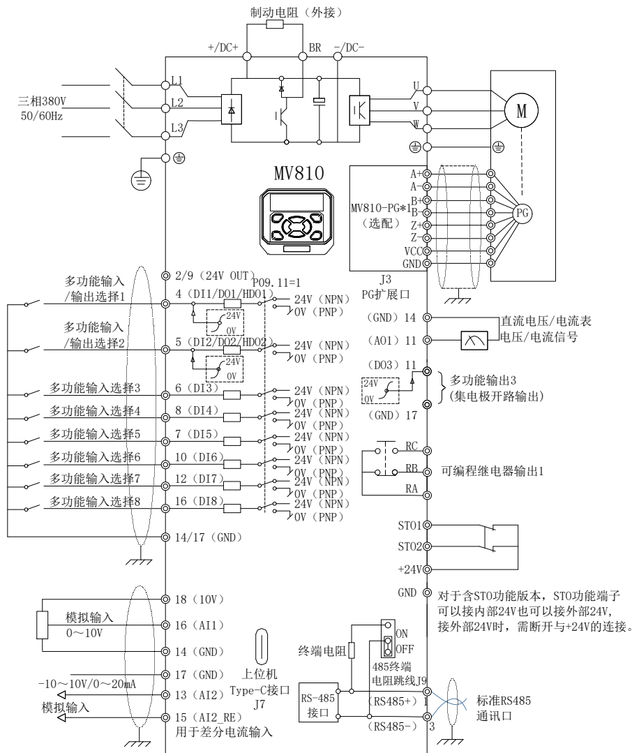
图 4-3 基本配线图 1
