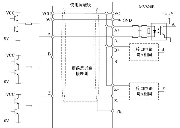
图 4-21 推挽信号 PG 接线示意图
