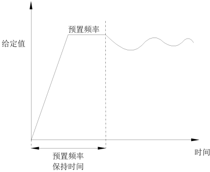
图7-46 PID预置频率运行示意图
