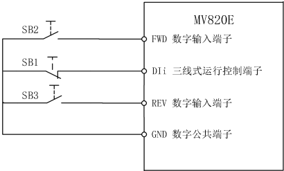
图7-20 三线式运转模式1
