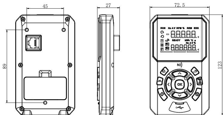
图2-25 大型远程LED键盘/操作面板（单位：mm）
