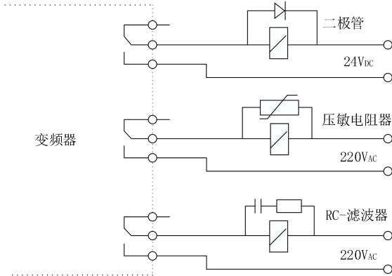
图 4-33 继电器、接触器及电磁制动器要求
