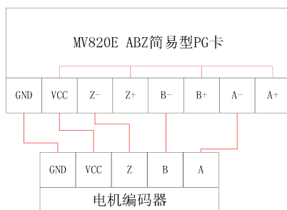
图 10-1 OC 接法
