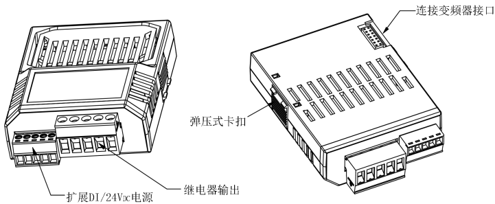
图2-5 端子部件示意图
