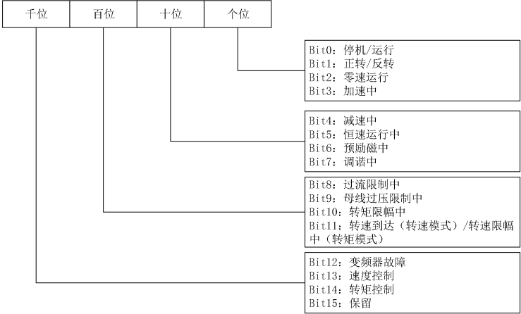
图7-2 变频器运行状态
