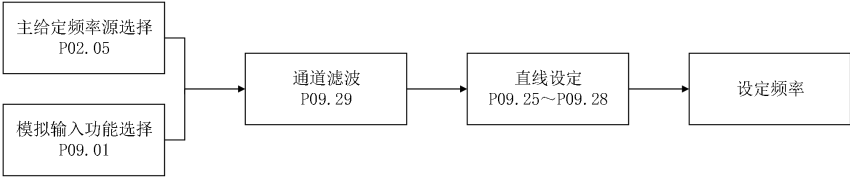
图7-23 给定通道输入与设定频率的关系
