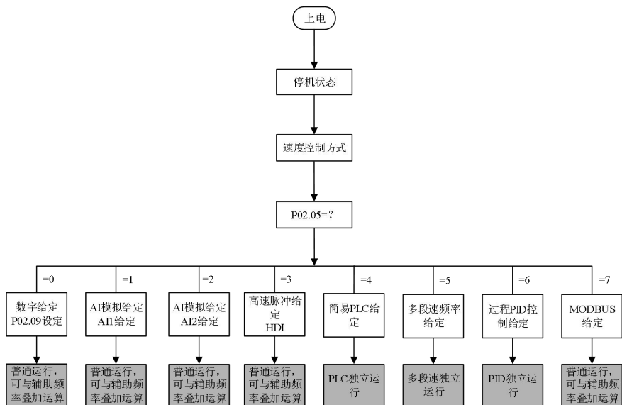
图 5-9 速度控制模式下运行方式选择
