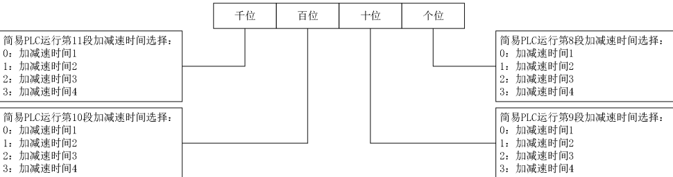
图7-41 简易PLC第8~11段加减速时间选择
