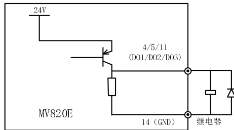
图 4-18 多功能输出端子 D0 接线方式
