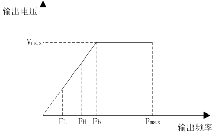
图7-6 极限频率参数定义示意图
