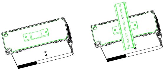
图2-18 轨道卡扣
