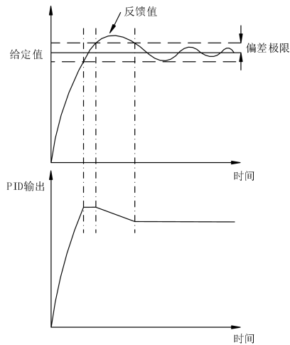
图7-44 偏差极限示意图
