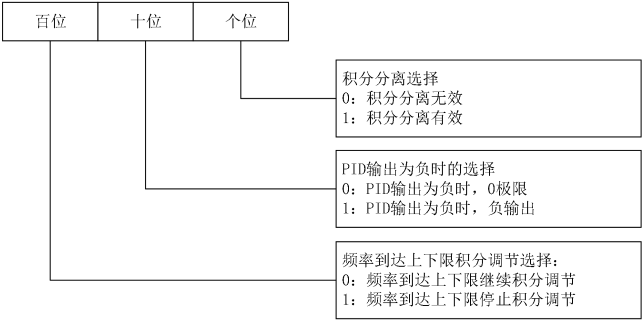
图7-45 PID输出特性选择
