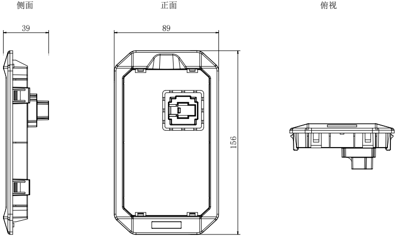
图2-21 大型键盘安装底座（单位：mm）
