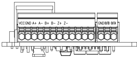
图2-7 端子丝印示意图
