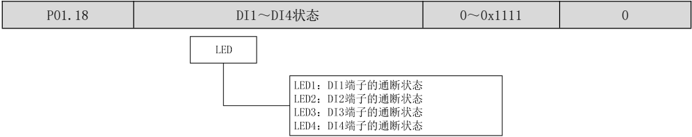
图7-3 开关量输入端子状态
