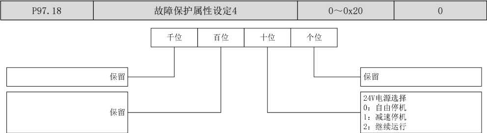
图7-56 故障保护属性设定4
