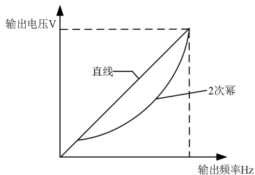
图 7-13 V/F 曲线
