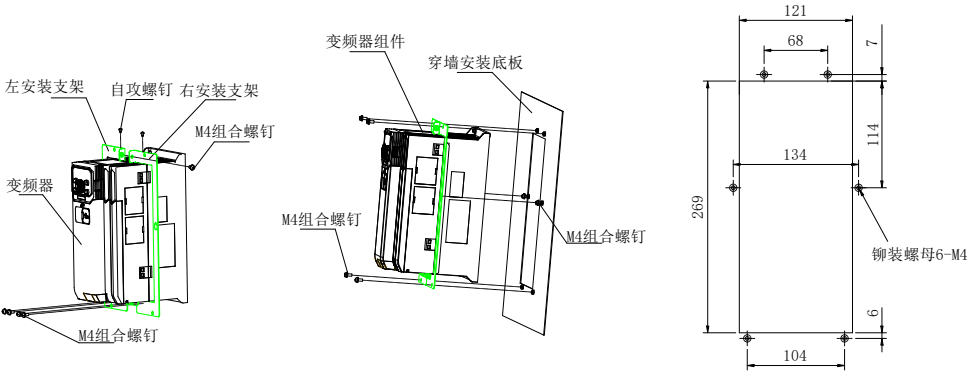
图2-14 MV810-EMBC嵌入式安装支架套料
