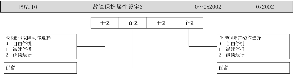
图7-54 故障保护属性设定2
