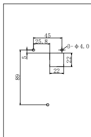
图a 开孔尺寸
