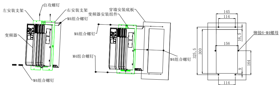
图2-15 MV810-EMBD嵌入式安装支架套料
