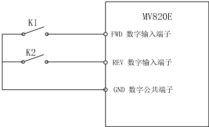
图7-19 两线式运转模式2
