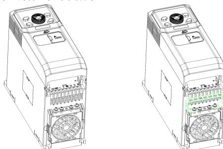
图2-17 绑线架
