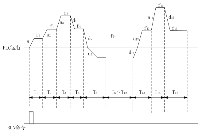
图7-36 PLC单循环后保持方式
