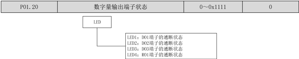
图7-5 开关量输出端子状态
