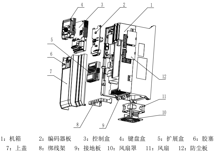
图 1-1 产品部分结构示意图 (以箱体 B 为例)
