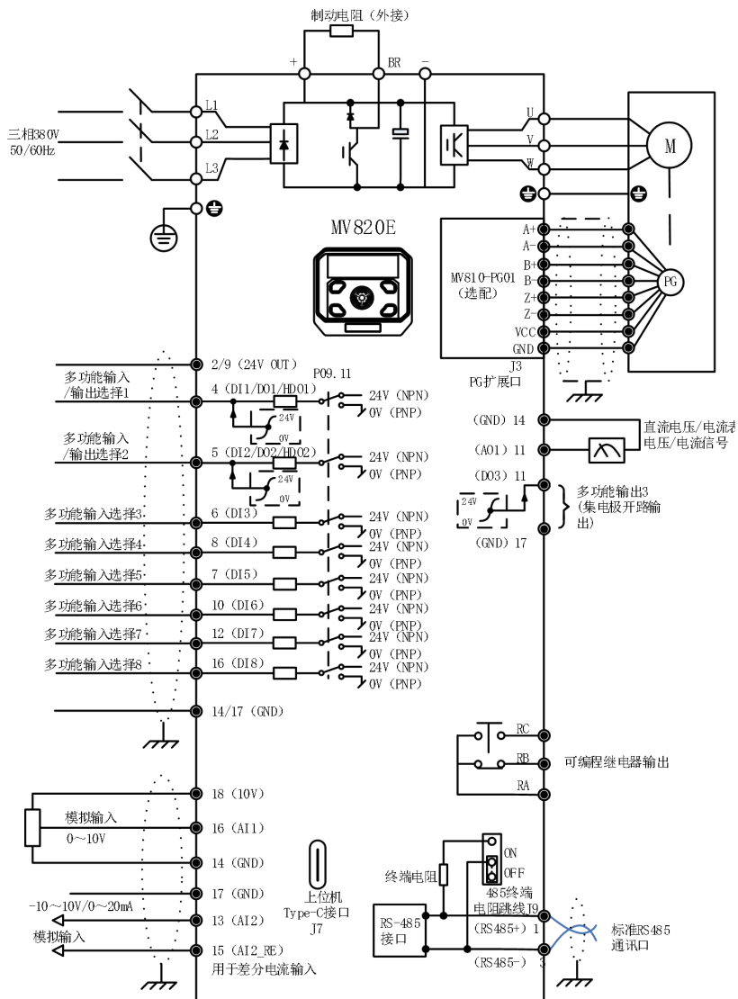
图 4-3 基本配线图
