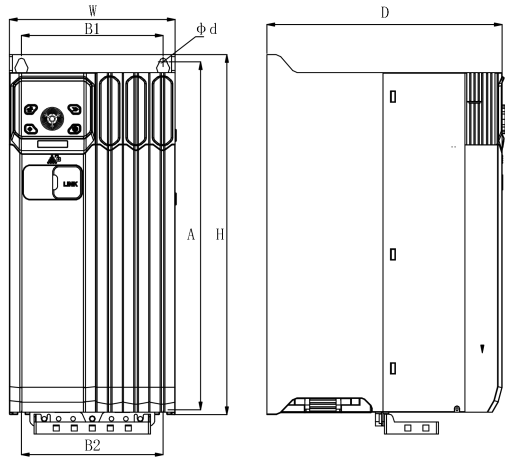
图 1-4 箱体 D
