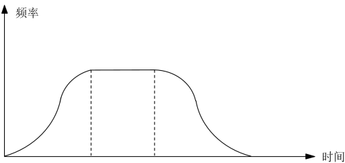
图7-26 S曲线加减速
