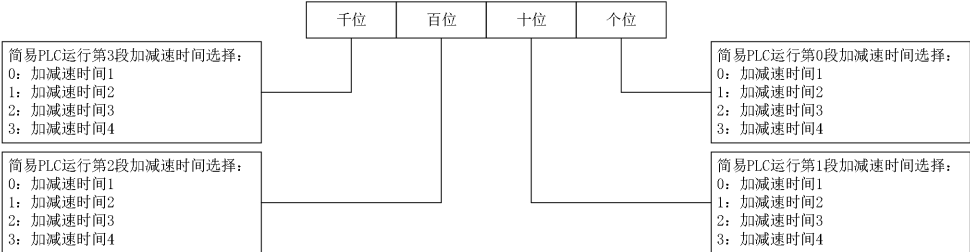
图7-39 简易PLC第0~3段加减速时间选择
