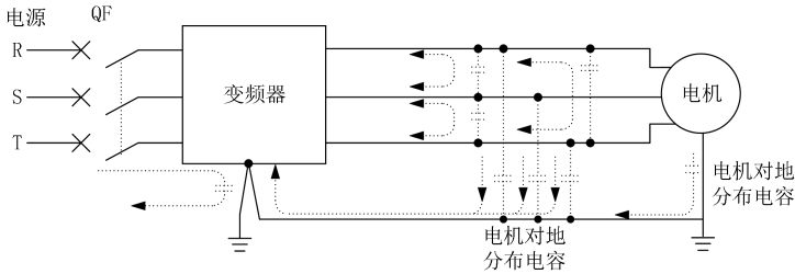
图 4-34 漏电流路径
