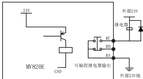
图 4-19 继电器输出端子 RA/RB/RC 接线方式
