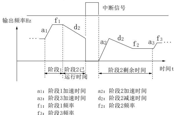
图7-38 PLC起动方式2
