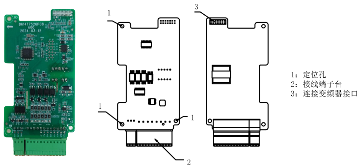
图2-6 外形及端子部件示意图
