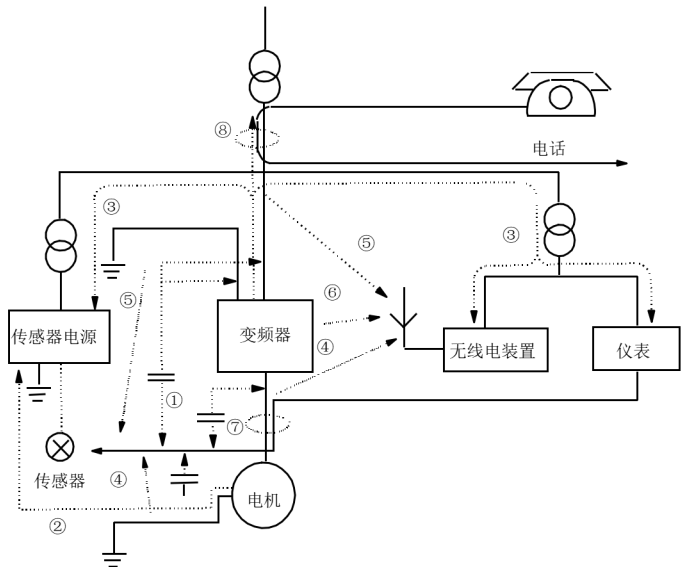
图 4-25 噪声传播路径示意图
