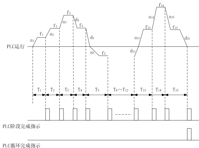
图7-33 简易PLC运行图
