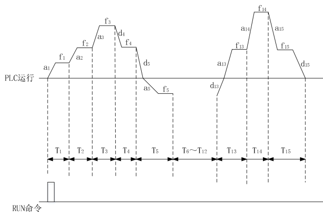
图7-35 PLC单循环后停机方式
