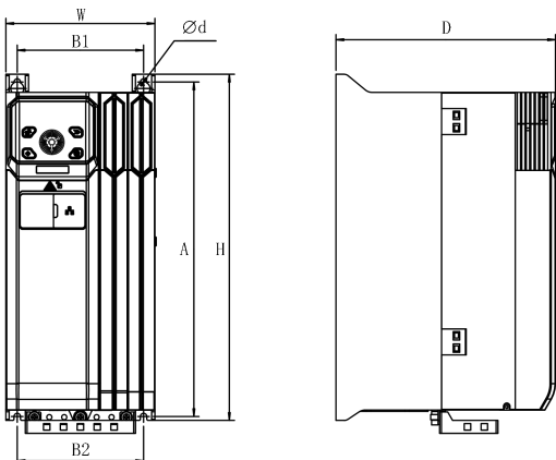
图 1-3 箱体 C
