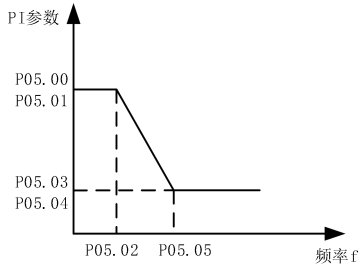
图7-9 PI参数示意图
