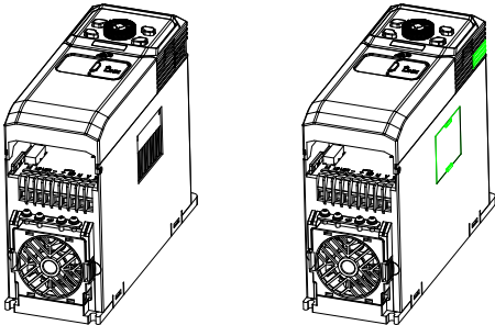
图2-12 防尘盖
