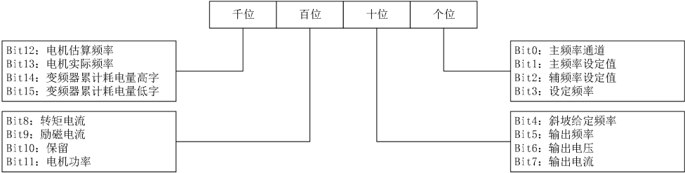
图7-47 LED运行显示参数选择1设定
