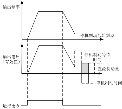
图7-16 减速停车+直流制动示意图
