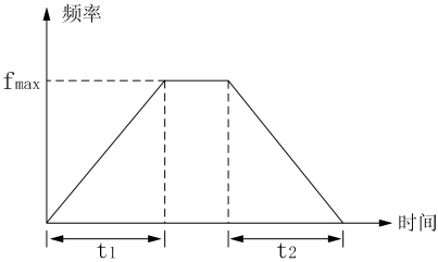
图7-25 直线加减速
