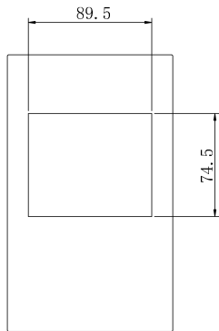
图2-20 操作面板固定座安装孔尺寸（单位：mm）
