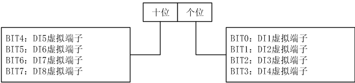
图7-22 虚拟输入端子设定
