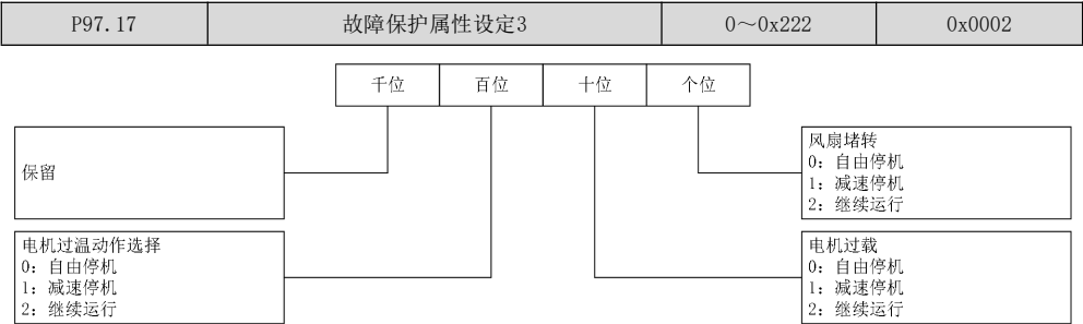
图7-55 故障保护属性设定3
