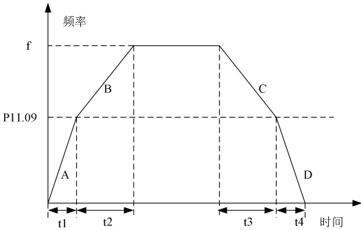
图7-28 加减速时间1、2切换示意图
