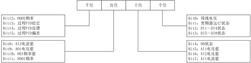
图7-48 LED运行显示参数选择2设定
