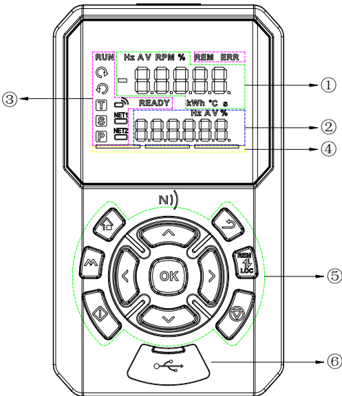
图 5-2 多功能键使用方法
