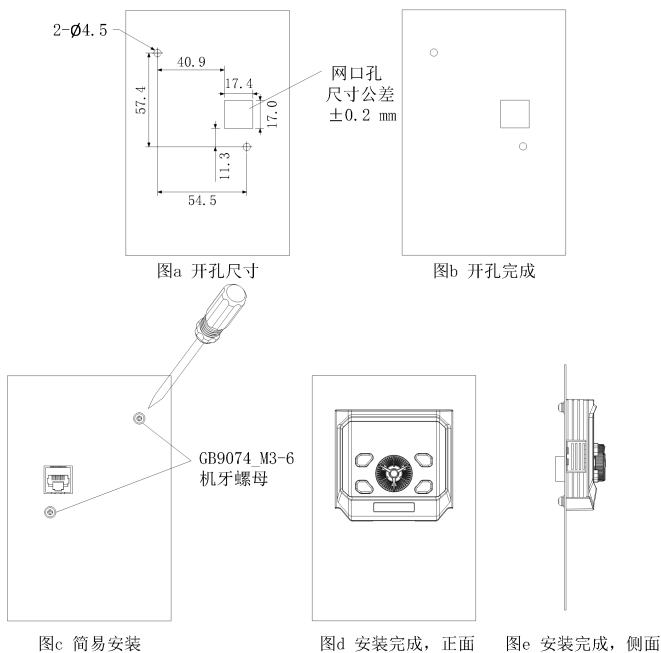
图2-24 远程LED键盘/操作面板简易安装方法
