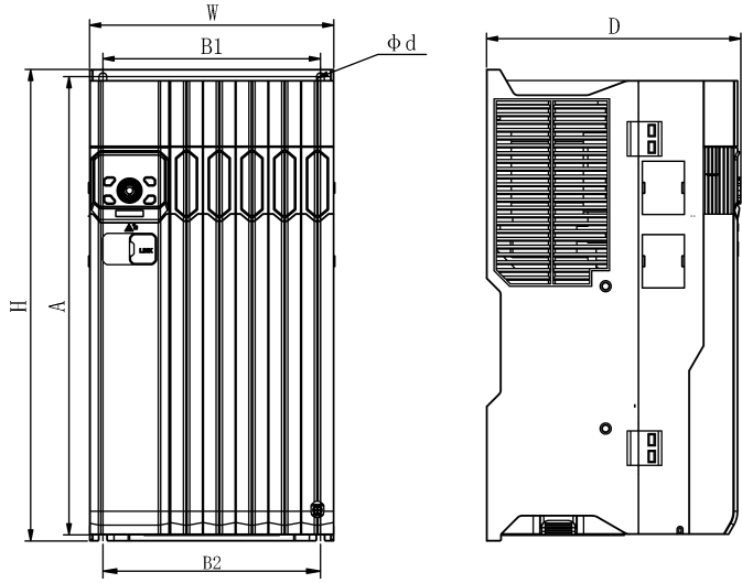
图 1-6 箱体 F
