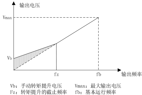
图7-15 转矩提升（提升量为阴影部分）
