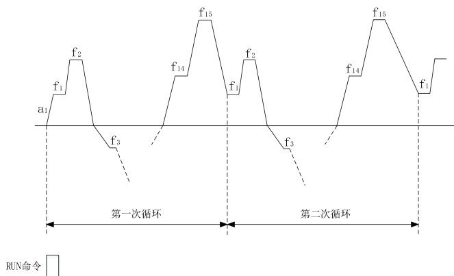
图7-37 PLC连续循环方式
