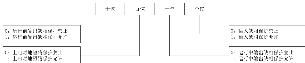
图7-52 输入、输出缺相保护设定
