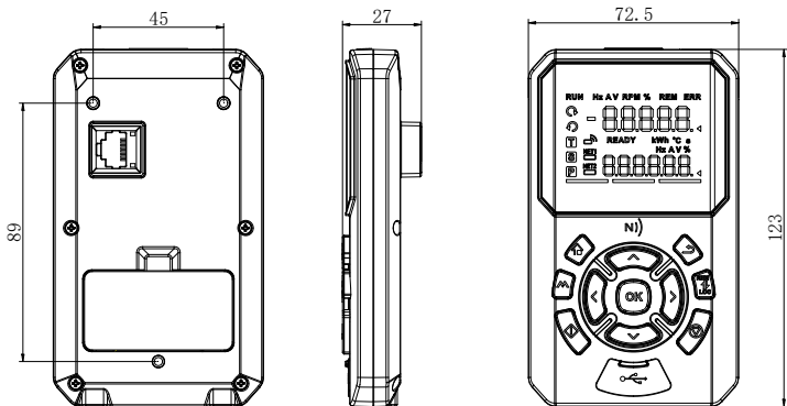
图 1-9 MV820-DP02 操作面板的外形和安装尺寸（单位：mm）
