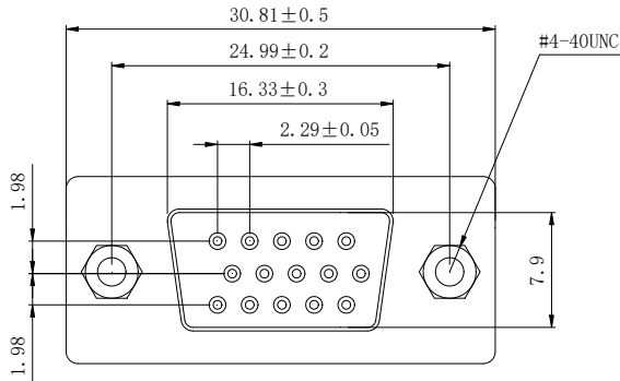
图2-9 MV820E-PG-S DB15示意图
