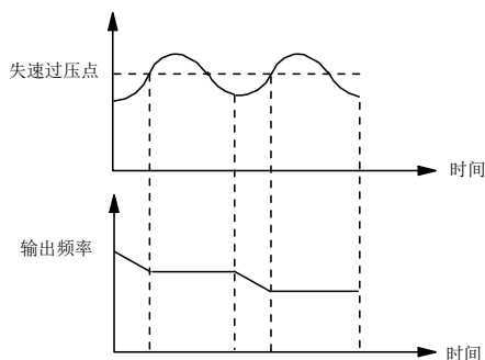
图7-51 过压失速功能
