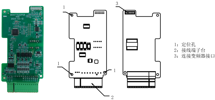
图2-8 外形及端子部件示意图
