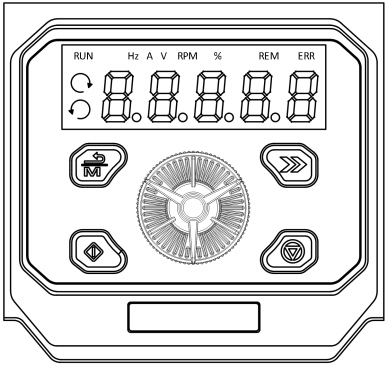
图 5-1 操作面板示意图
