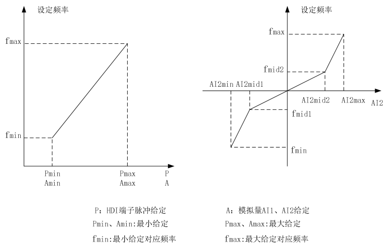
图7-24 模拟输入频率特性曲线
