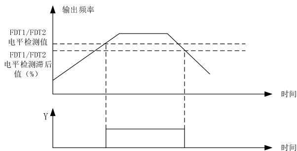
图7-32 频率水平检测示意图
