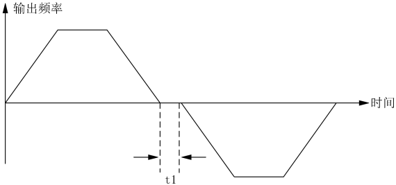
图7-17 正反转死区时间
