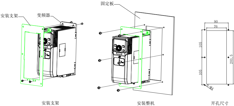
图2-13 MV810-EMBB嵌入式安装支架套料
