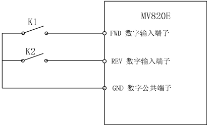
图7-18 两线式运转模式1
