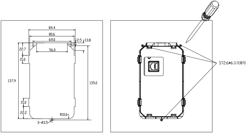
图2-22 大型操作面板固定座安装孔尺寸（单位：mm）
