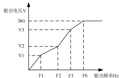
图 7-14 多点 V/F 曲线
