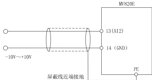
图 4-7 端子电压单端输入配线图
