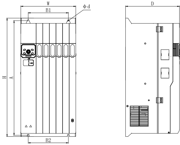
图 1-7 箱体 G
