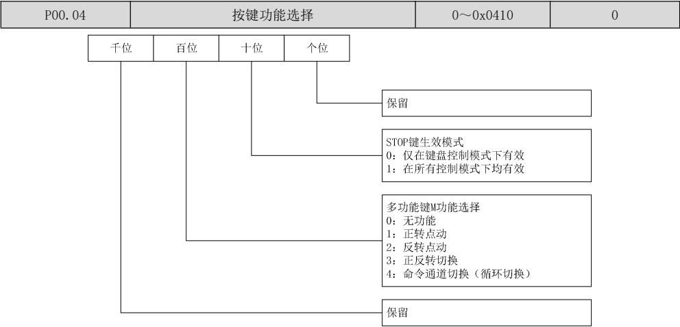
图7-1 按键功能选择
