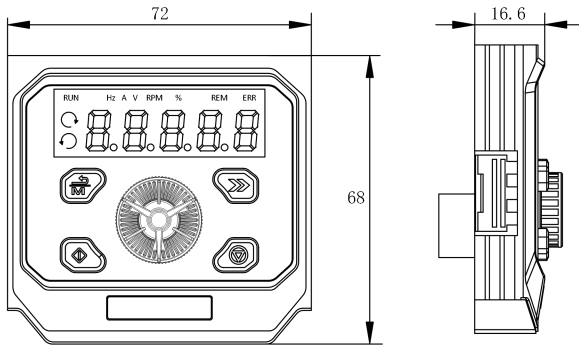
图 1-8 MV820-DP01 操作面板的外形和安装尺寸（单位：mm）
