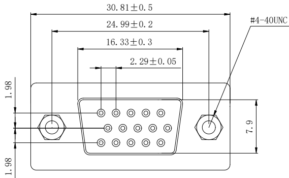
图2-11 MV820E-PG-F DB15示意图
