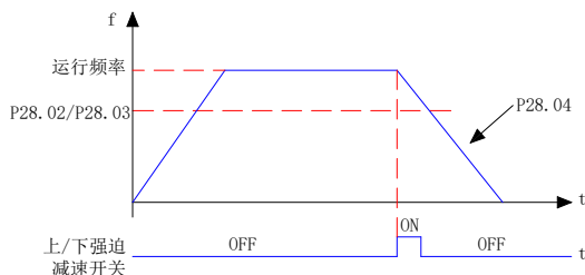
图7-49 强迫减速运行原理
