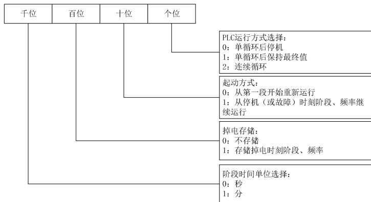
图7-34 简易PLC运行方式选择
