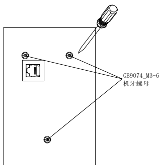
图c 简易安装
