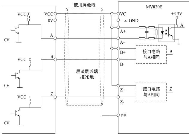
图 4-20 集电极开路信号 PG 接线示意图
