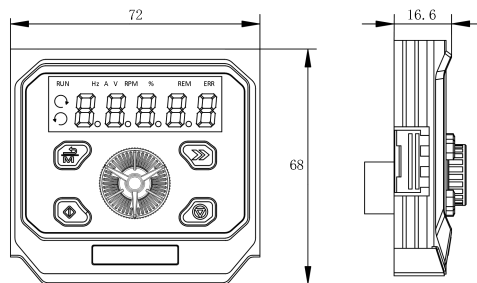
图2-23 远程LED键盘/操作面板
