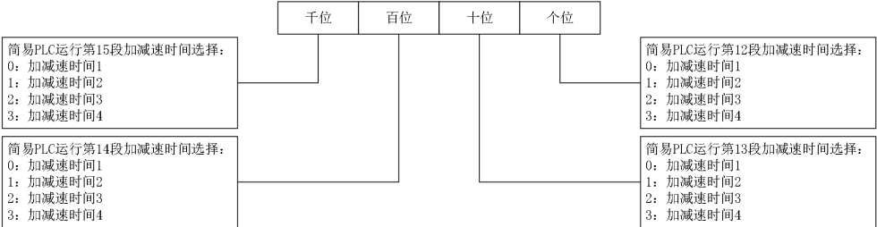
图7-42 简易PLC第12~15段加减速时间选择
