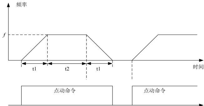
图7-29 点动运行参数说明
