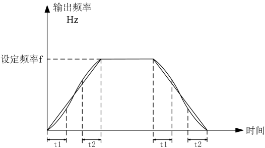
图7-27 S曲线开始、结束段时间比例
