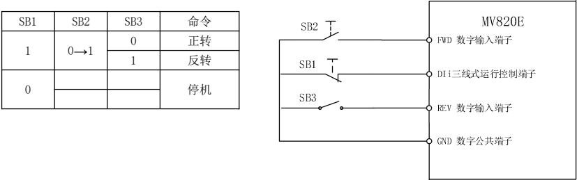
图7-21 三线式运转模式2
