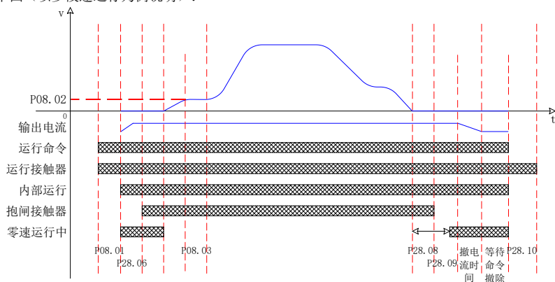
图7-50 运行时序图
