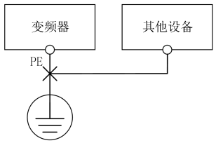
图 4-32 接地示意图 4
