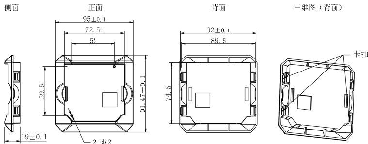
图2-19 键盘安装底座（单位：mm）
